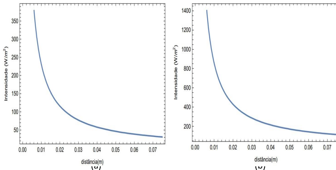
FIGURA 4. Intensidade de radiação UV: (a) sem reflexão e (b) com reflexão 73%
