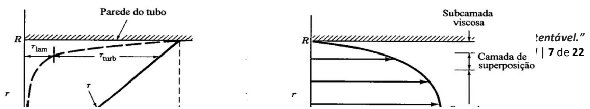
FIGURA 3. Estrutura do escoamento em um tubo: (a) tensão de cisalhamento e (b) velocidade média.
