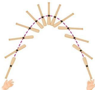
Figura 12 - Movimento do centro de massa
