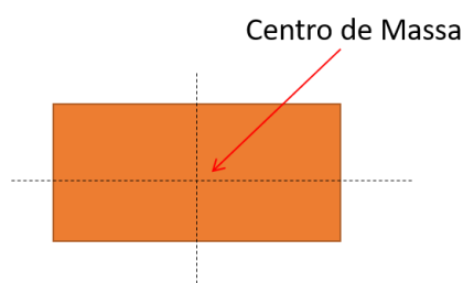
Figura 13 – Centro de massa de uma placa
