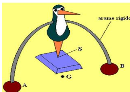
Figura 11 - Movimento do centro de massa.
