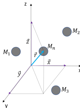
Figura 15 - Centro de massa de um sistema de partículas no espaço.
