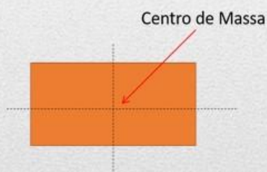
Figura 12: Centro de Massa de uma placa Fonte: Elaborado pelo autor, 2020.
