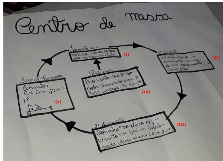
Figura 27 - Modelo matemático elaborado pela Equipe 3 para analisar o experimento sobre o equilíbrio da ponte de Da Vinci.
