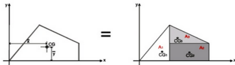
Figura 13 a) – Centro de massa de uma placa
